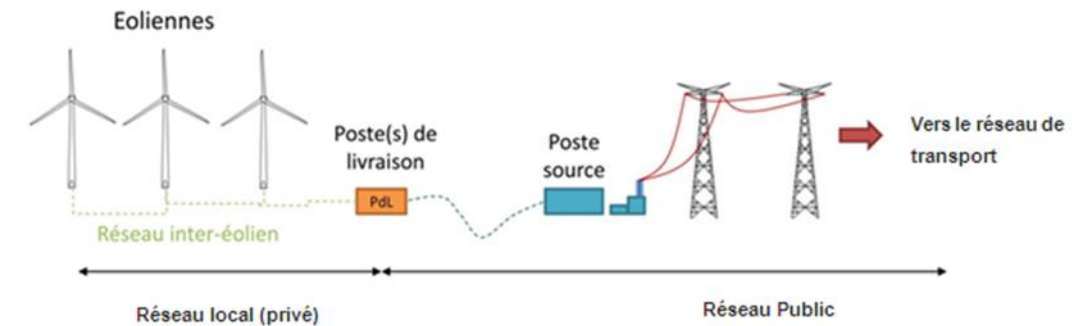
Figure 24 : Schéma de raccordement électrique d'un parc éolien
