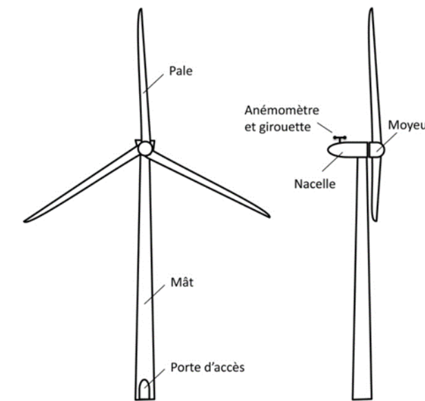
Figure 21 : Schéma simplifié d'un aérogénérateur
