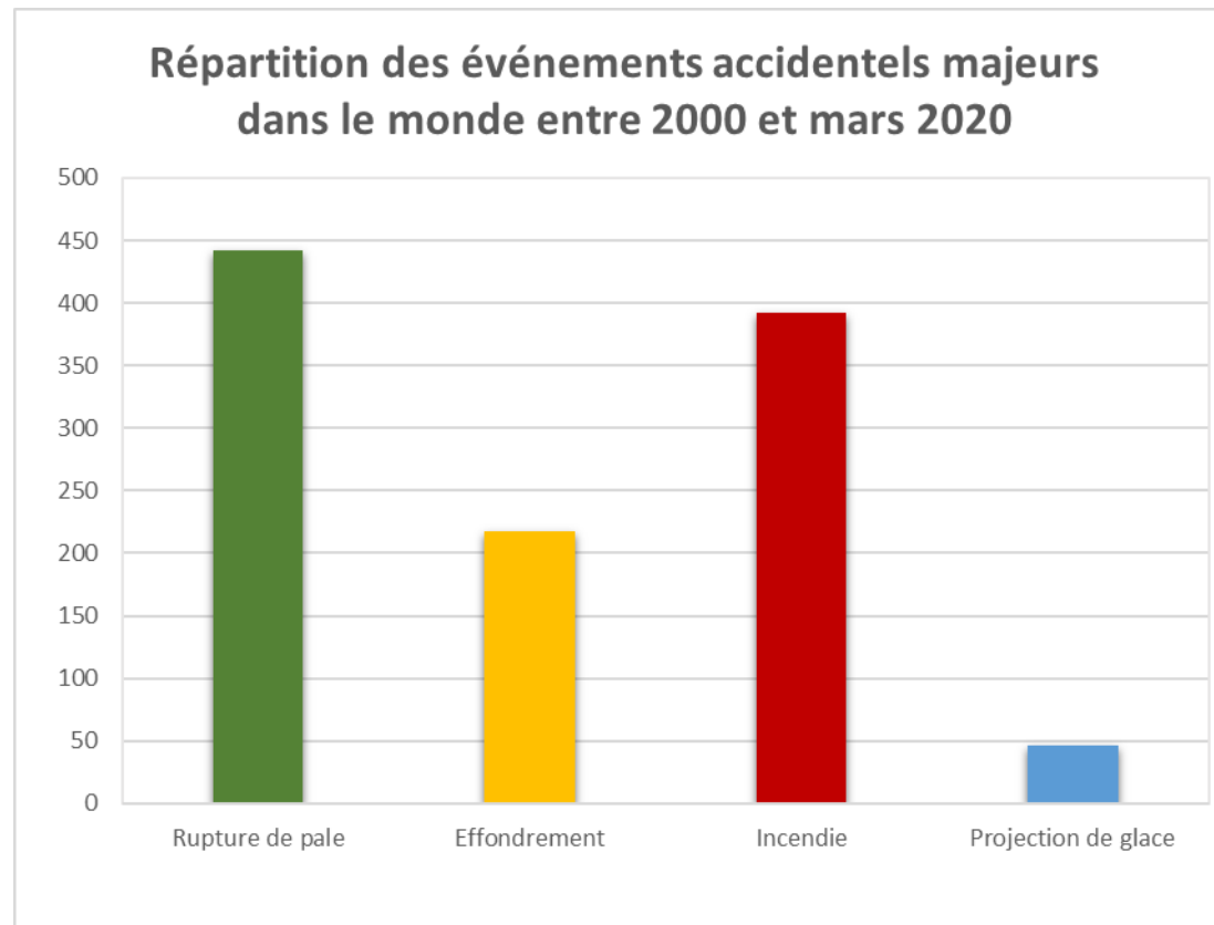
Figure 26 : Répartition des événements accidentels majeurs dans le monde entre 2000 et mars 2020
