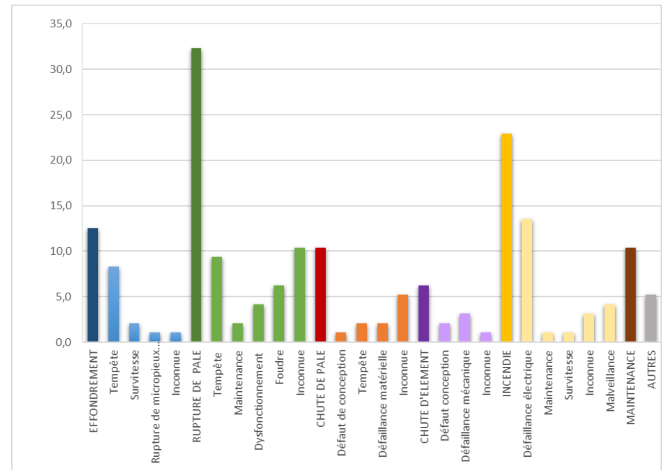
Figure 25 : Répartition des événements accidentels et de leurs causes premières sur le parc d'aérogénérateurs français entre 2000 et juin 2020
