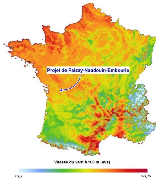
Figure 16 : Vitesse moyenne du vent à 100 m (Source : à partir des données GWA-Vortex-WAsP)
