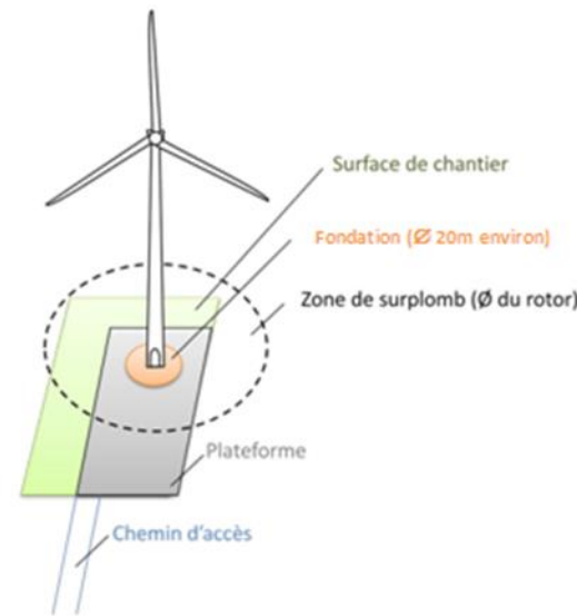
Figure 22 : Illustration des emprises au sol d'une éolienne
