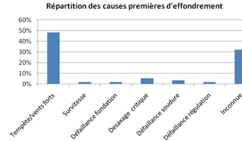
Figure 27: Répartition des causes premières d'effondrement
