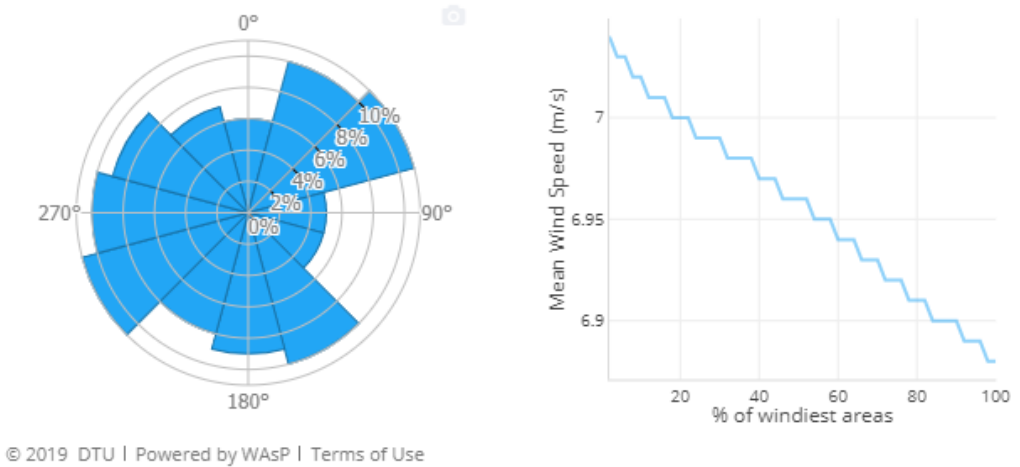
Figure 17 : Rose des vents et fréquence par vitesse à 100 m au niveau du projet éolien des Chaumes (Source : GWA, WAsP)
