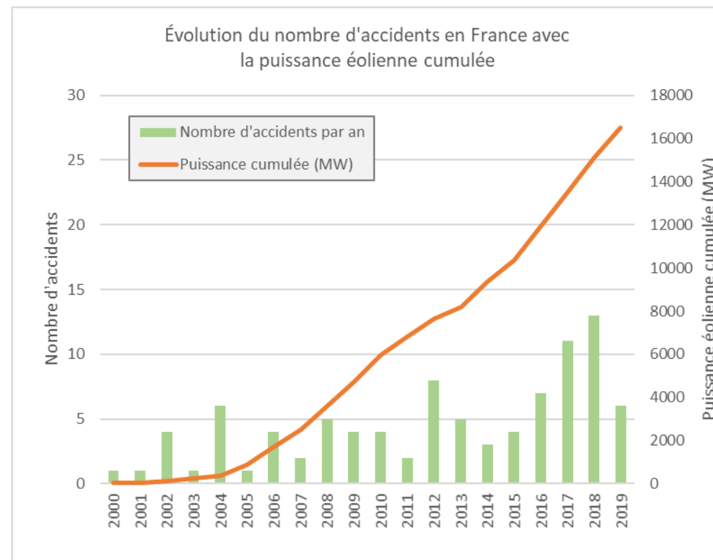
Figure 30 : Evolution du nombre d'incidents annuels en France et puissance éolienne installée 1
