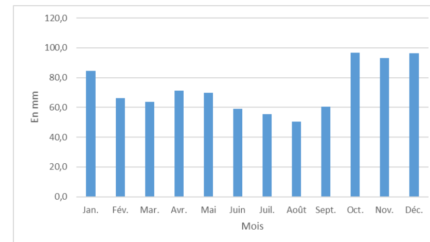
Figure 14 : Hauteurs mensuelles en mm des précipitations à Niort (Source : Météo France)
