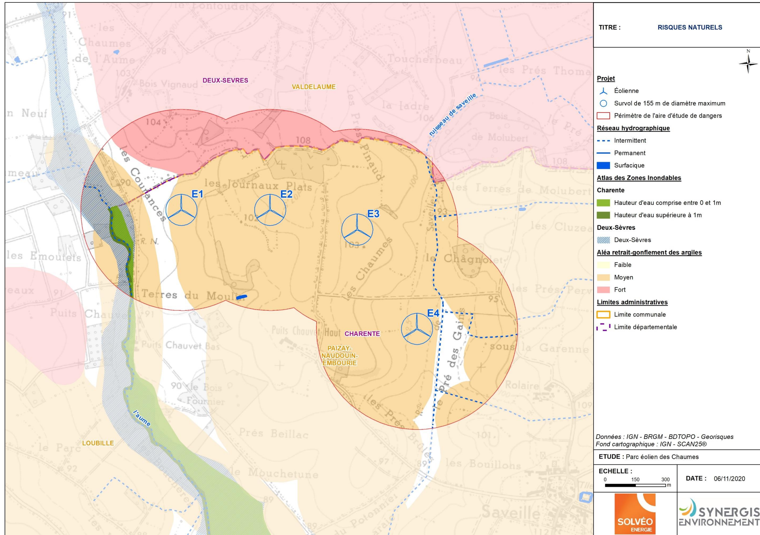
Figure 19 : Risques naturels identifiés sur l'aire d'étude de dangers
