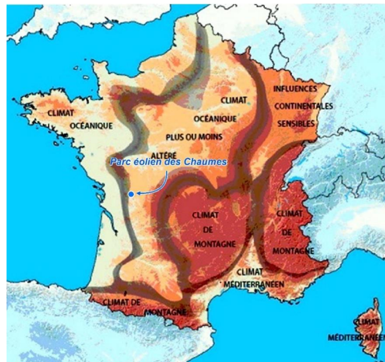
Figure 12 : Les zones climatiques en France et la localisation de l'aire d'étude de dangers du projet des Chaumes (Source : Météo-France)
