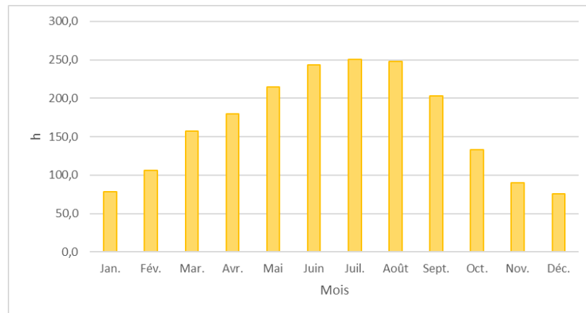
Figure 15 : Ensoleillement moyen par mois à Niort en nombre d'heures (Source : Météo France)
